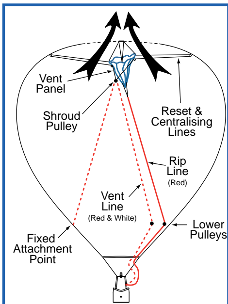
• Smart Vent - centre pull mode
