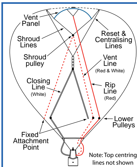
• Lite Vent - parachute mode
