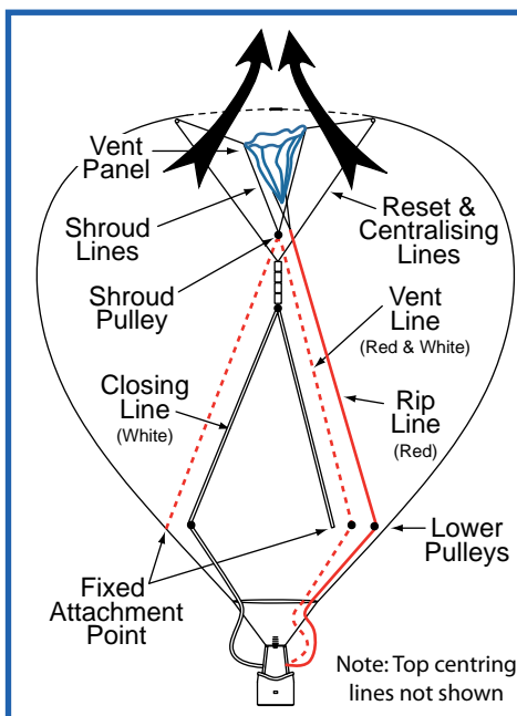
• Lite Vent - centre pull mode
